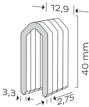
WZK Klammer Durchmesser 3,3 mm Länge 40 mm
